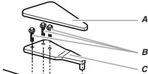
A. Tapa de la bisagra superior B. Tornillos de cabeza hexagonal de la bisagra de 5/16" C. Bisagra superior
