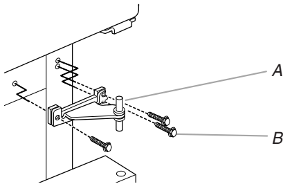
A. Bisagra central B. Tornillos para bisagra de cabeza hexagonal de \frac{5}{16} "
