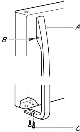
A. Manija del congelador B. Tornillo de ajuste de 1/4" C. Tornillos de cabeza plana de la manija
