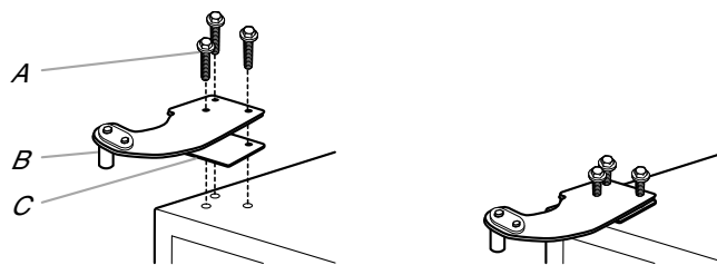
A. Tornillos para bisagra de cabeza hexagonal de \frac{5}{16} " B. Pasador de la bisagra superior C. Espaciador de plástico
